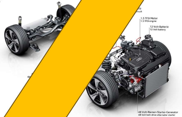
Audi A3 Mild-Hybrid 48 Volt-Antriebsstrang Mild hybrid 48 volt drivetrain 03/24
